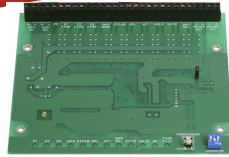
Ancillary PCB VF1822-x0
